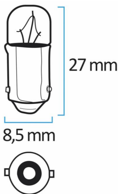
LÁMPARA, PILOTO DE MATRÍCULA REF... 050110 CAJA 10 UDS
